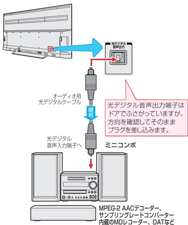
【本機背面】
