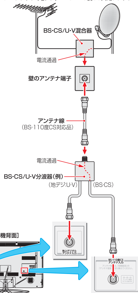
UHFアンテナ(地デジ) BS・110度CS共用アンテナ
